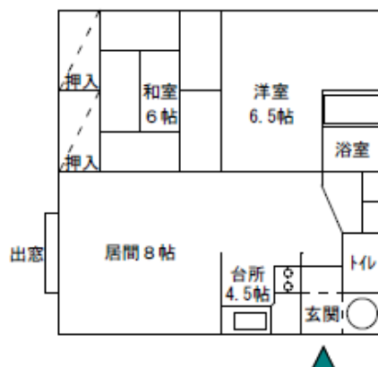
2階3号平面図
