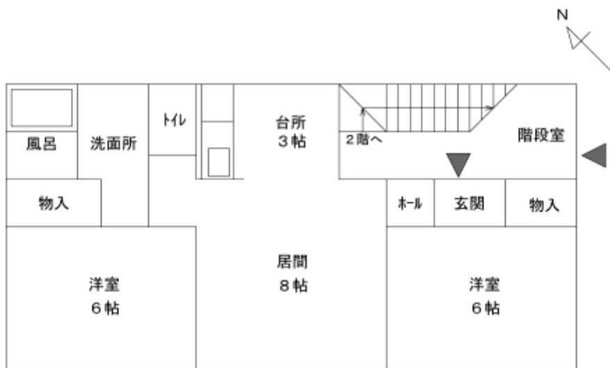
1階平面図
