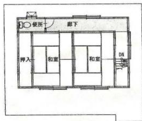
2階平面図
