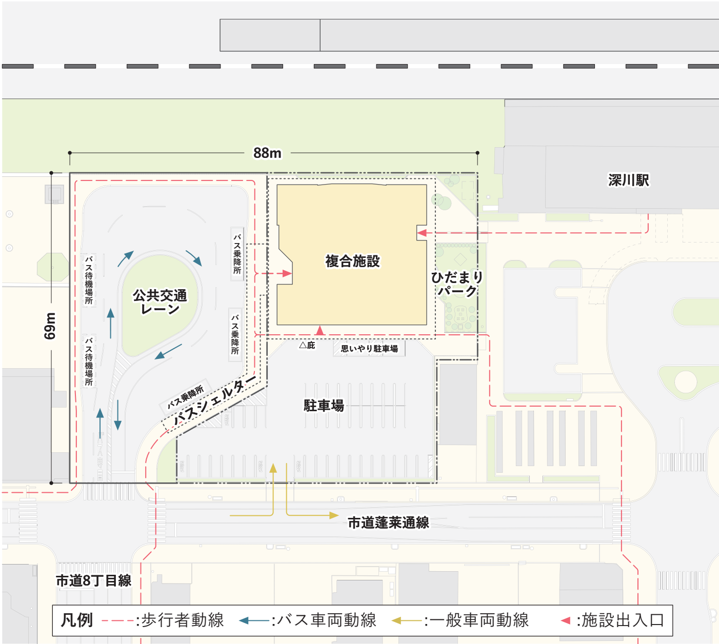
配置図
