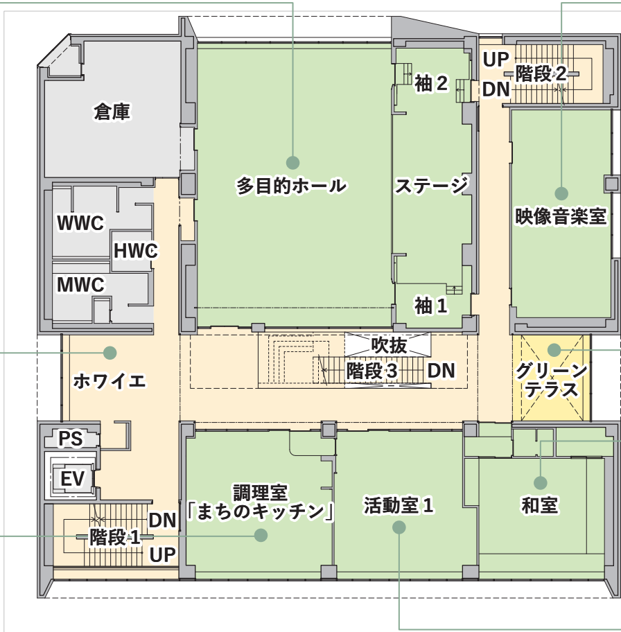
[ 2 階平面図 ]
