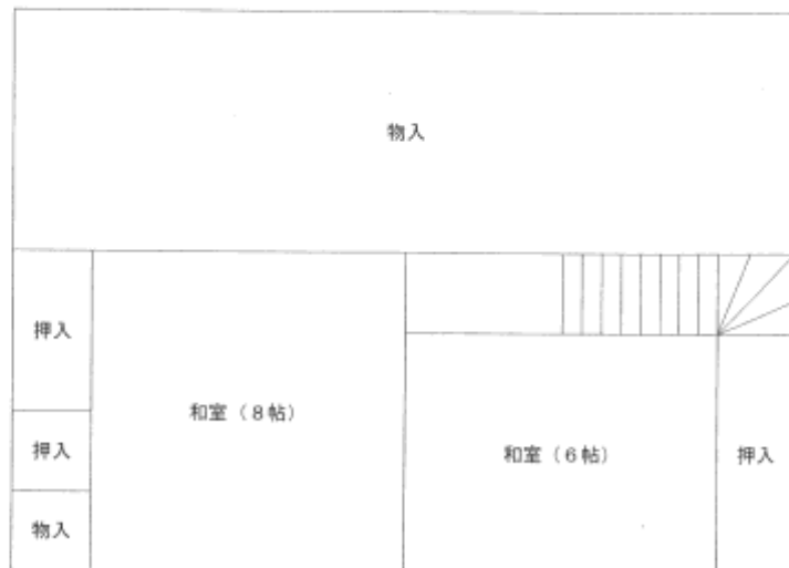
2階平面図
