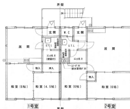
2階平面図
