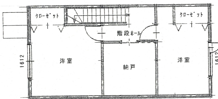
2階平面図
