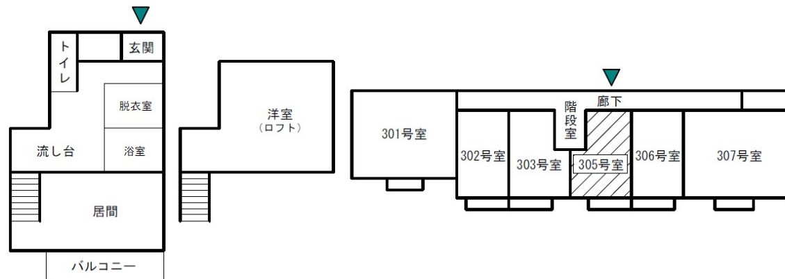
3階305号平面図
