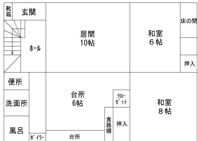
1 階平面図
