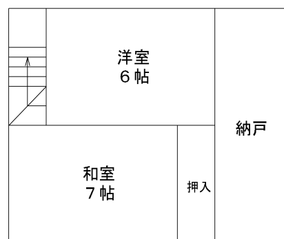
2 階平面図
