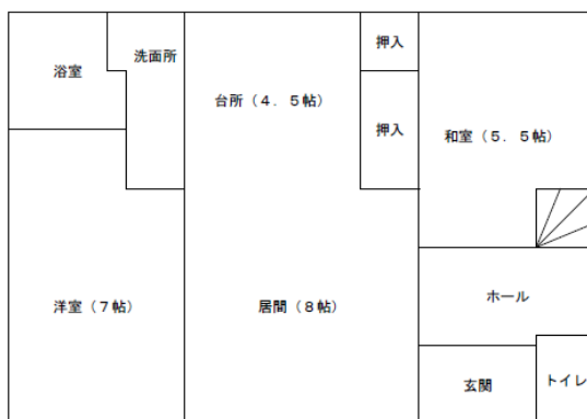
1階平面図
