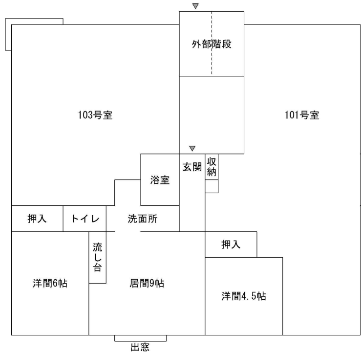
102号室 平面図
