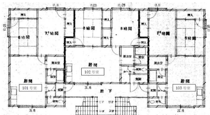
平面図（間取図）
