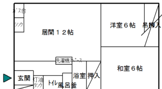
2階202号平面図
