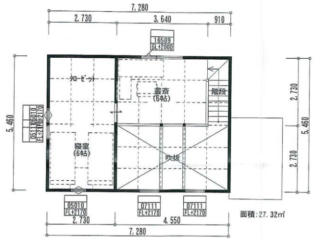
2階平面図
