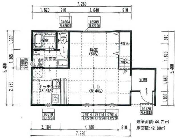
1階平面図
