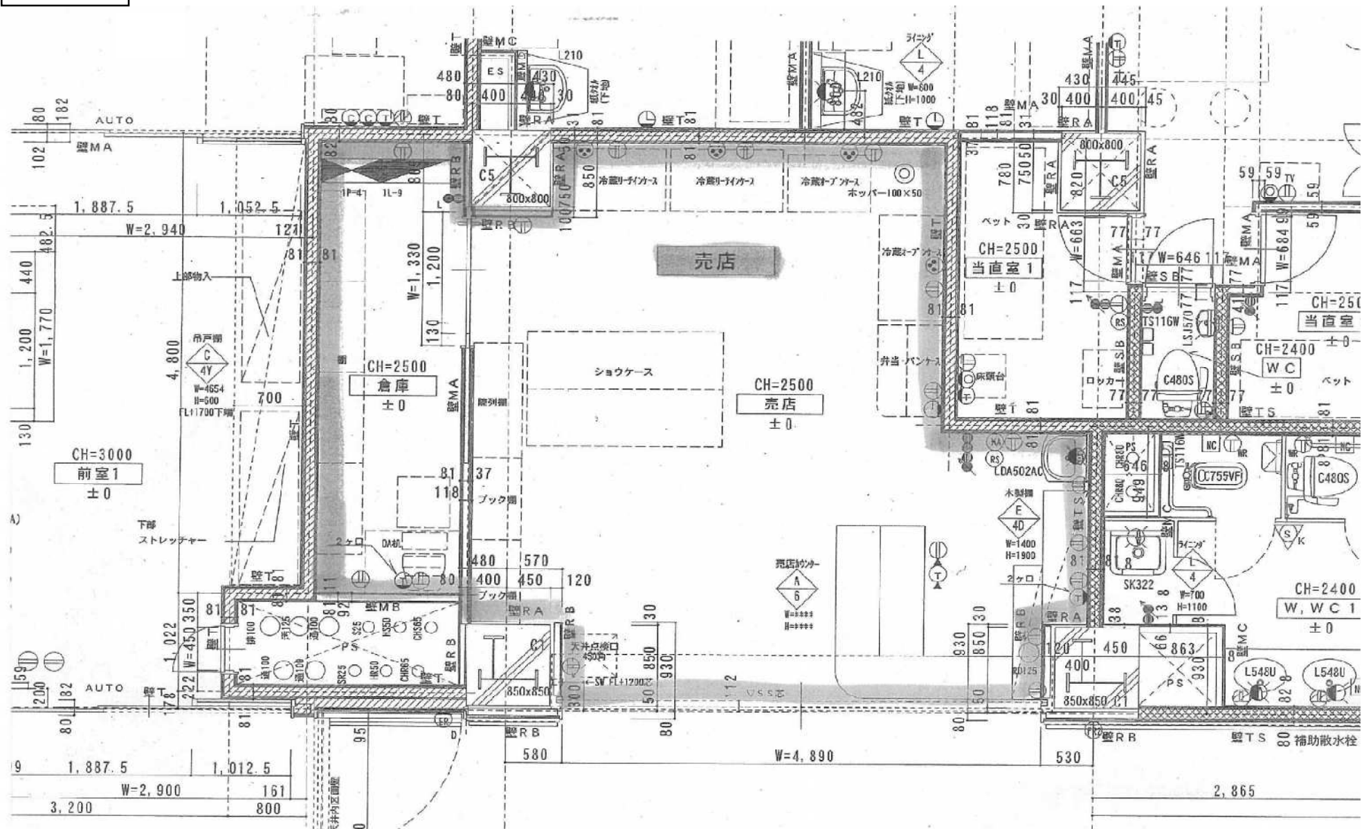
売店平面図
